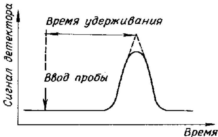
Рис.5. Определение времени удерживания по хроматографическому пику.
