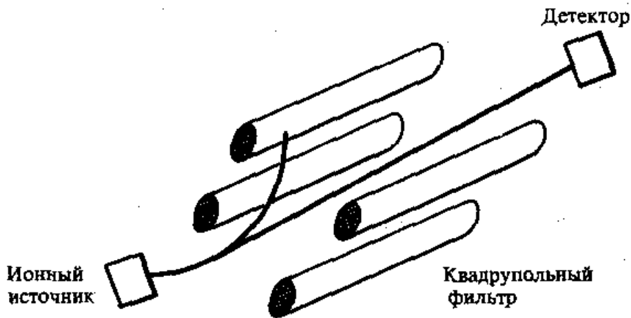
Рис.7. Схема устройства квадрупольного масс-спектрометра.
