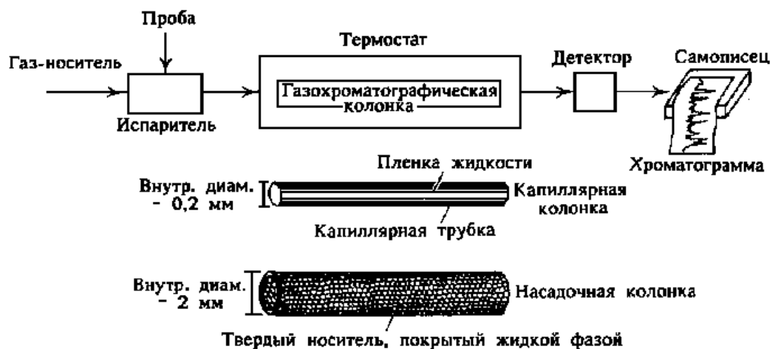
Рис.2. Схема газового хроматографа.
