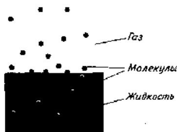
Рис.1. Адсорбция на границе раздела жидкой и газовой фаз.
