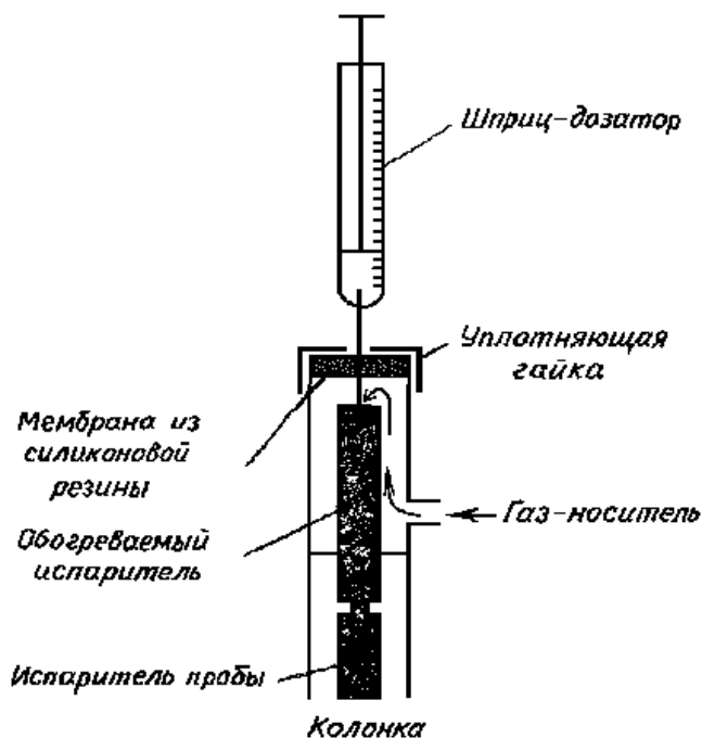
Рис.3. Введение пробы шприцем-дозатором через самоуплотняющуюся резиновую прокладку.
