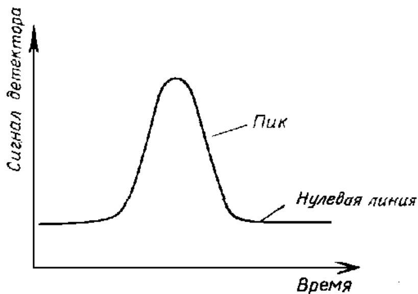
Рис.4. Изменение высоты хроматографического пика во времени.
