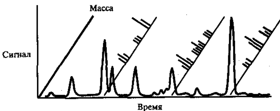
Рис.11. Пример хроматограммы по всем ионам.
